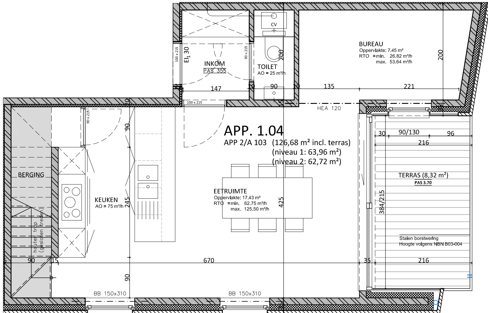
1e VERDIEPING
