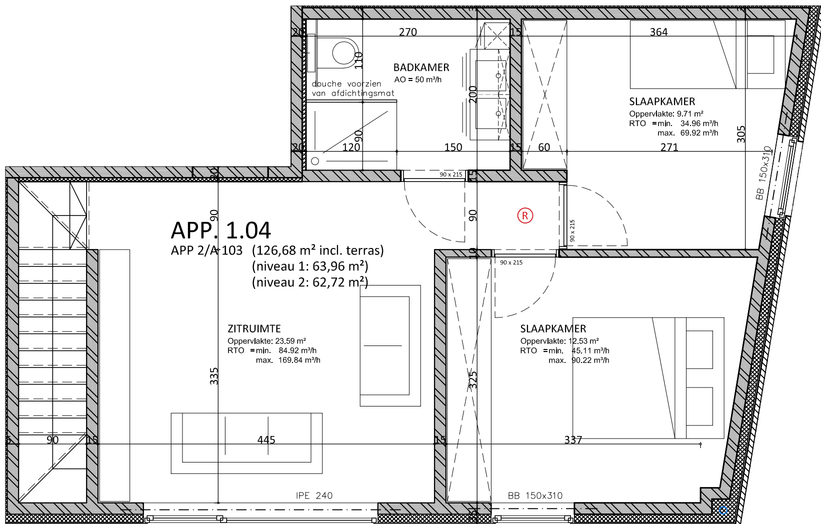
2e VERDIEPING
