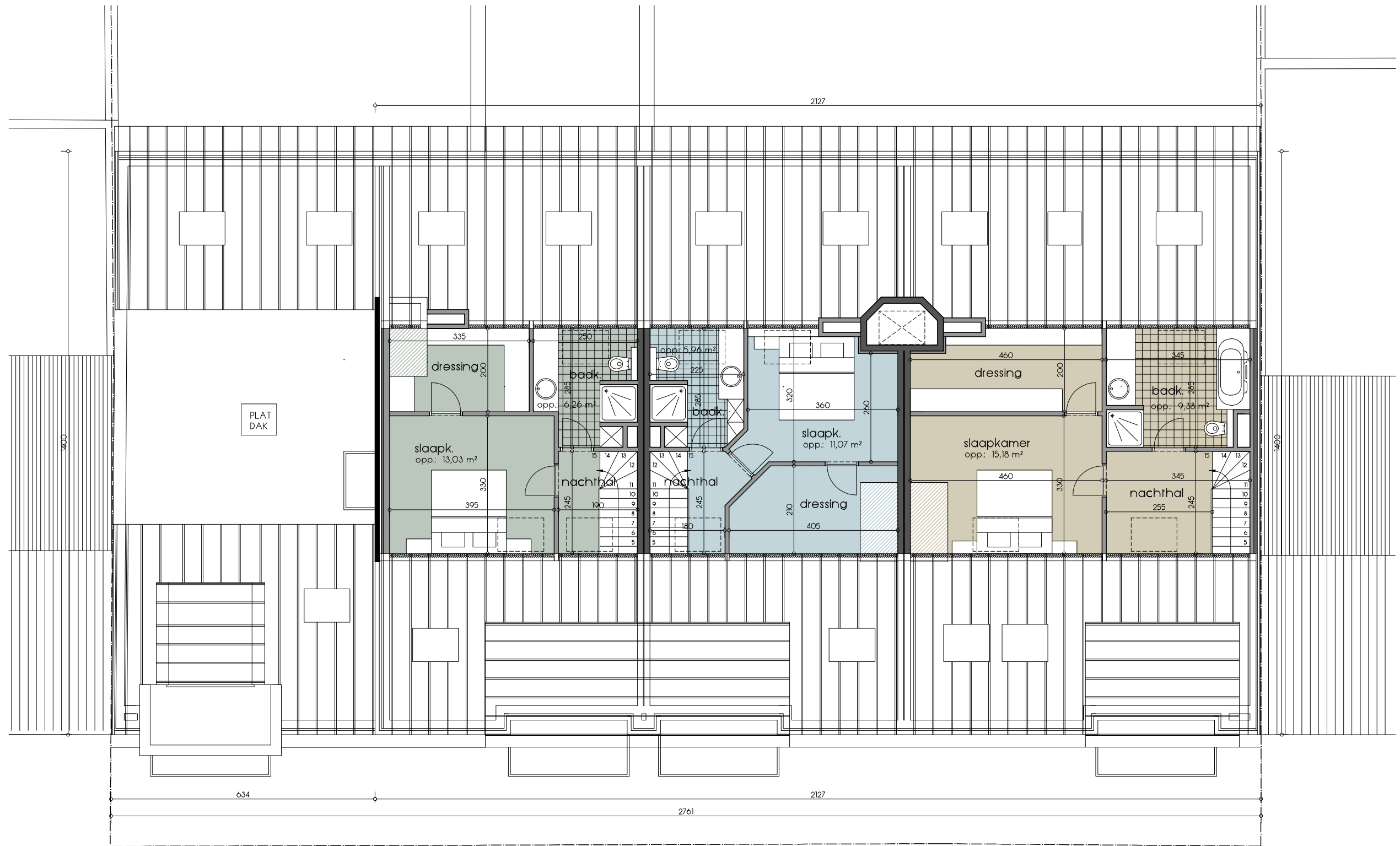
dakverdieping 2
